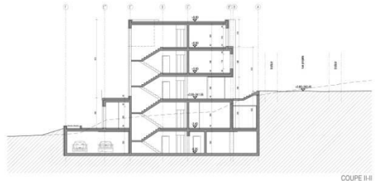
COUPE II-II
