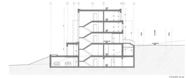
COUPE III-III
